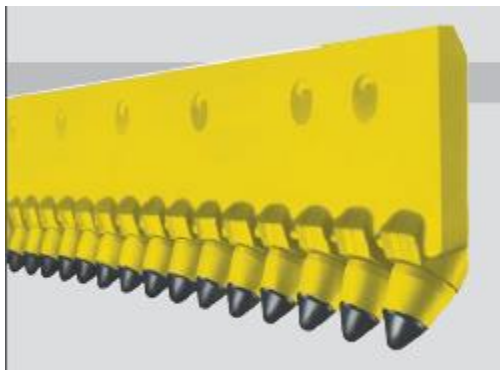
Solda na Frente + Barra de Carbetto no meio
