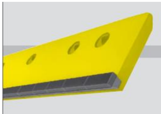
Placa grande + barra de Carbetto
